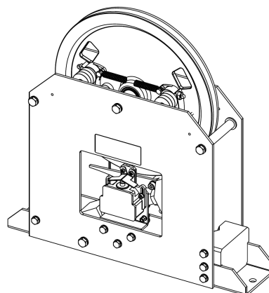
Limitatore di velocità unidirezionale mod. R12BF Unidirectional overspeed governor type R12BF Limiteur de vitesse unidirectionnel mod. R12BF Einseitig gerichteter Geschwindigkeitsbegrenzer Typ R12BF Limitador de velocidad unidireccional mod. R12BF
