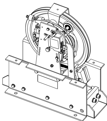
Limitatore di velocità unidirezionale mod. R10BF Unidirectional overspeed governor type R10BF Limiteur de vitesse unidirectionnel mod. R10BF Einseitig gerichteter Geschwindigkeitsbegrenzer Typ R10BF Limitador de velocidad unidireccional mod. R10BF
