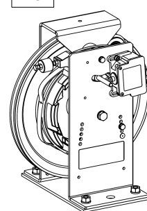
Abb. 2 Geschwindigkeits- begrenzer Typ R5 / R5S / R6. Andere Fußausführung möglich.
