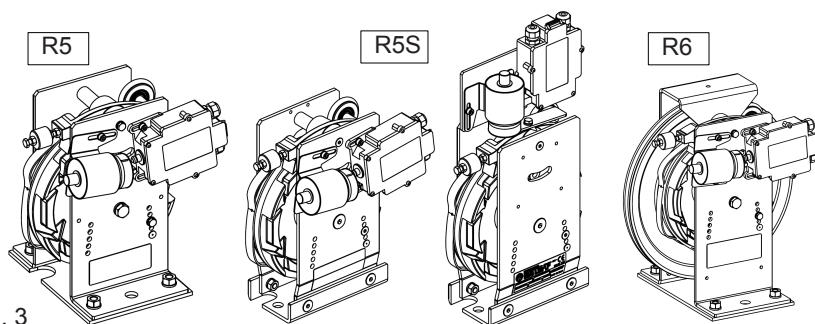
Fig. 3 Limitatori di velocità Mod. R5-R5S-R6 con comando a distanza.
