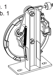
Fig. 1 Limitador de velocidad mod. R3
