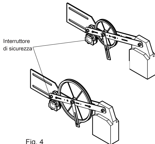
Fig. 4 Tenditore con contrappeso orizzontale completo di interruttore di sicurezza
