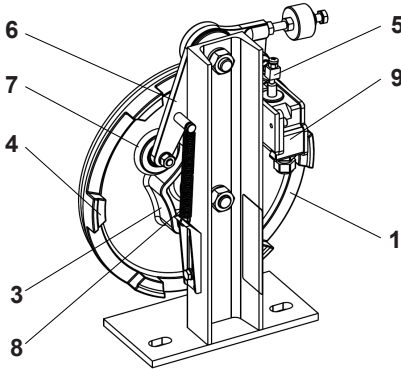
Abb. 1 Geschwindigkeitsbegrenzer Typ R3
