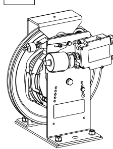
Abb. 3 Geschwindigkeits- begrenzer Typ R5 / R5S / R6 Fernauslösung Andere Fußausführung möglich.
