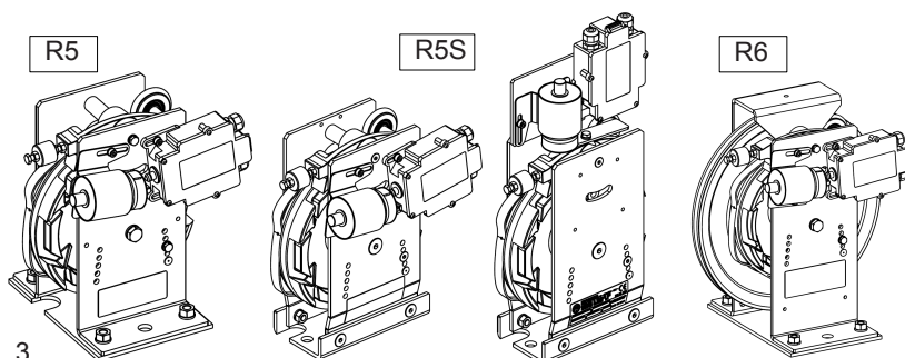
Fig. 3 Limitor de velocidad Mod. R5-R5S-R6 con mando a distancia.
