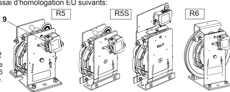
Fig. 2 Limiteur de vitesse mod. R5-R5S-R6 sans commande à distance.
