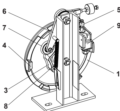
Fig. 1 Limitador de velocidad mod. R3
