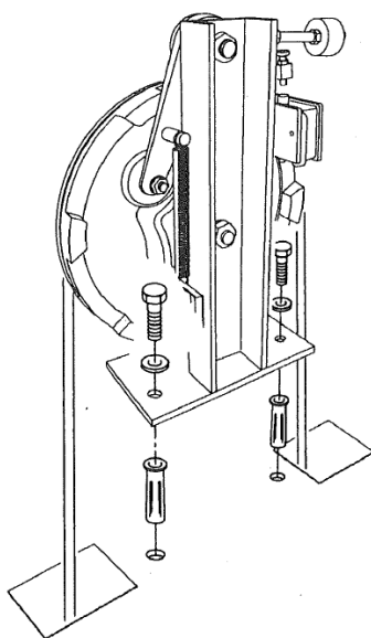
Рис. 1 Ограничитель скорости Моды. R3
