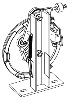
Рис. 1 Ограничитель скорости модели R3.
