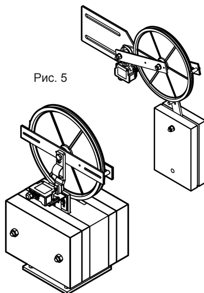
Рис. 5 Натяжитель с вертикальным противовесом, для направляющей и натяжения троса с предохранительным выключателем, версия с креплением в пол или с креплением к руководству.
