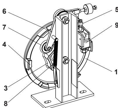
Рис. 1 Ограничитель скорости модели R3
