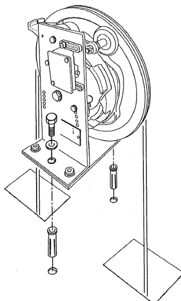
Рис. 2 Ограничитель скорости Моды. R5-R5S-R6
