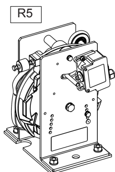
Рис. 2 Ограничитель скорости, модели R5 / R5S / R6 без устройства дистанционного управления; возможные версии с другими носителями.
