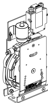
Рис. 3 Ограничитель скорости, модели R5 / R5S / R6 с устройством дистанционного управления; возможные версии с другими носителями.
