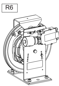
Рис. 3 Ограничитель скорости, модели R5 / R5S / R6 с устройством дистанционного управления; возможные версии с другими носителями.
