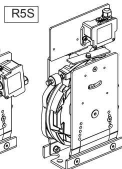
Рис. 2 Ограничитель скорости, модели R5 / R5S / R6 без устройства дистанционного управления; возможные версии с другими носителями.
