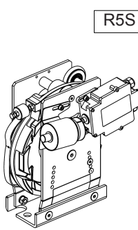
Рис. 3 Ограничитель скорости, модели R5 / R5S / R6 с устройством дистанционного управления; возможные версии с другими носителями.
