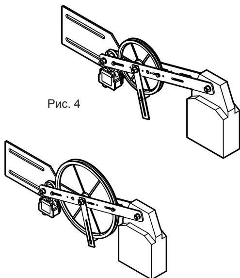
Рис. 4 Натяжитель устройства с горизонтальным противовесом, для направляющей и натяжения троса, с предохранительным выключателем.
