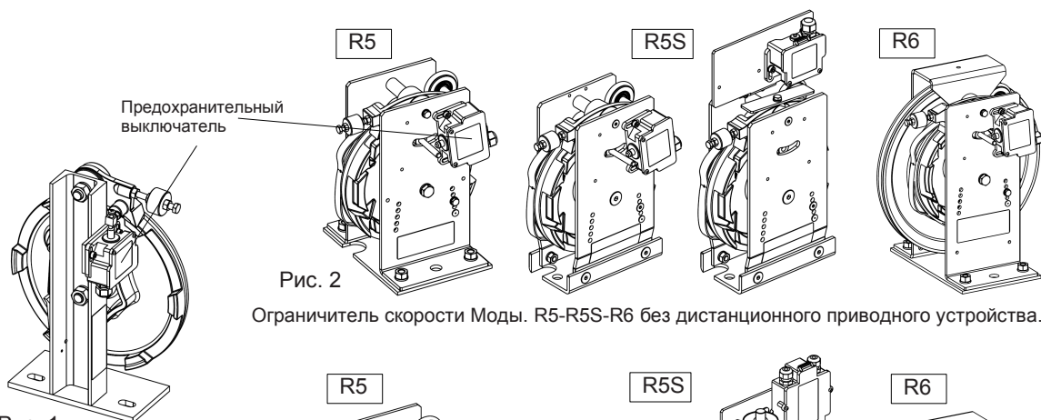
Рис. 1 Ограничитель скорости Моды. R3.
