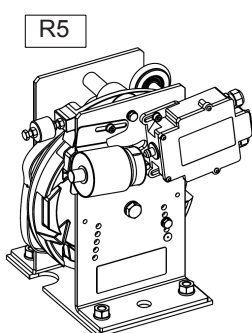
Рис. 3 Ограничитель скорости, модели R5 / R5S / R6 с устройством дистанционного управления; возможные версии с другими носителями.
