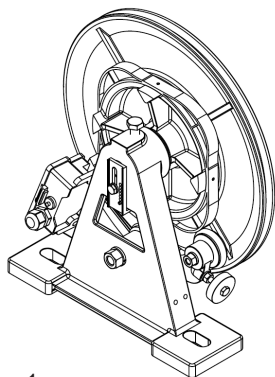
Рис. 1 Ограничитель скорости, модели R1LR - R1 - R1 200 - R1 250
