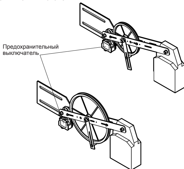
Рис. 2 Натяжитель с горизонтальным противовесом в комплекте с предохранительным выключателем.
