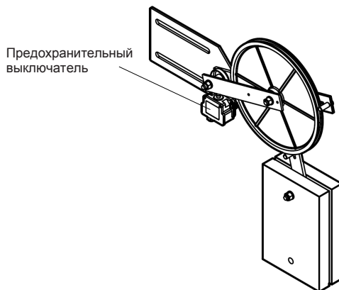
Рис. 4 Натяжитель с вертикальным противовесом с предохранительным выключателем. (Крепление к направляющей)
