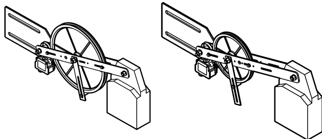
Рис. 2 Натяжитель устройства с горизонтальным противовесом, для направляющей и натяжения троса, с предохранительным выключателем.
