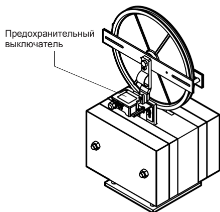
Рис. 3 Натяжитель с вертикальным противовесом с предохранительным выключателем
