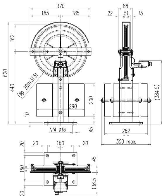
Моды. R4V Ø200-250-300
