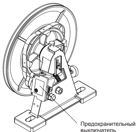
Рис. 1 Ограничитель скорости Моды. R1LR - R1 - R1 200 - R1 250
