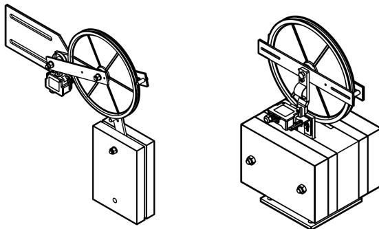
Рис. 3 Натяжитель с вертикальным противовесом, для направляющей и натяжения троса с предохранительным выключателем, версия с креплением в пол или с креплением к руководству.
