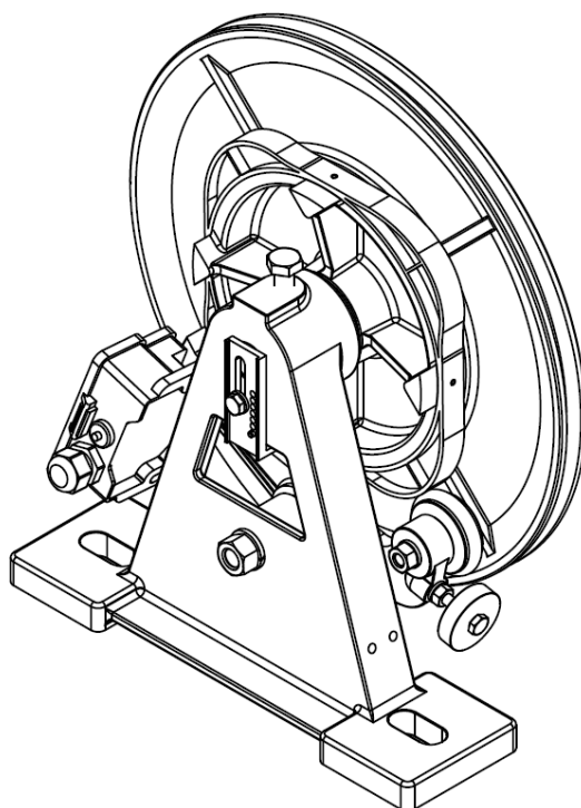
ОГРАНИЧИТЕЛЬ СКОРОСТИ R1LR – R1 – R1 200 – R1 250
